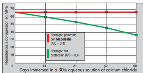
Fig. 4: Efecto del Mapelastíc ante el deterioro mecánico del hormigón debido a las sales de deshielo a base de cloruro de calcio
