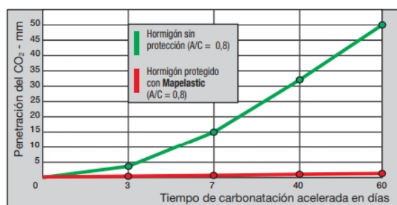
Fig. 2: Efecto del Mapelastic sobre la carbonatación acelerada (30% de \text{CO}_2 ) en un hormigón poroso
